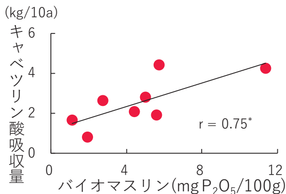
図 2-9 土壌のバイオマスリンとキャベツのリン酸吸収量との関係
